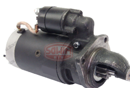
ROZRUSZNIK SILNIK: PERKINS 10 ZĘBÓW
